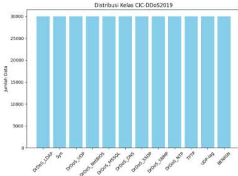
Gambar 3. Distribusi Kelas CIC-DDoS2019
